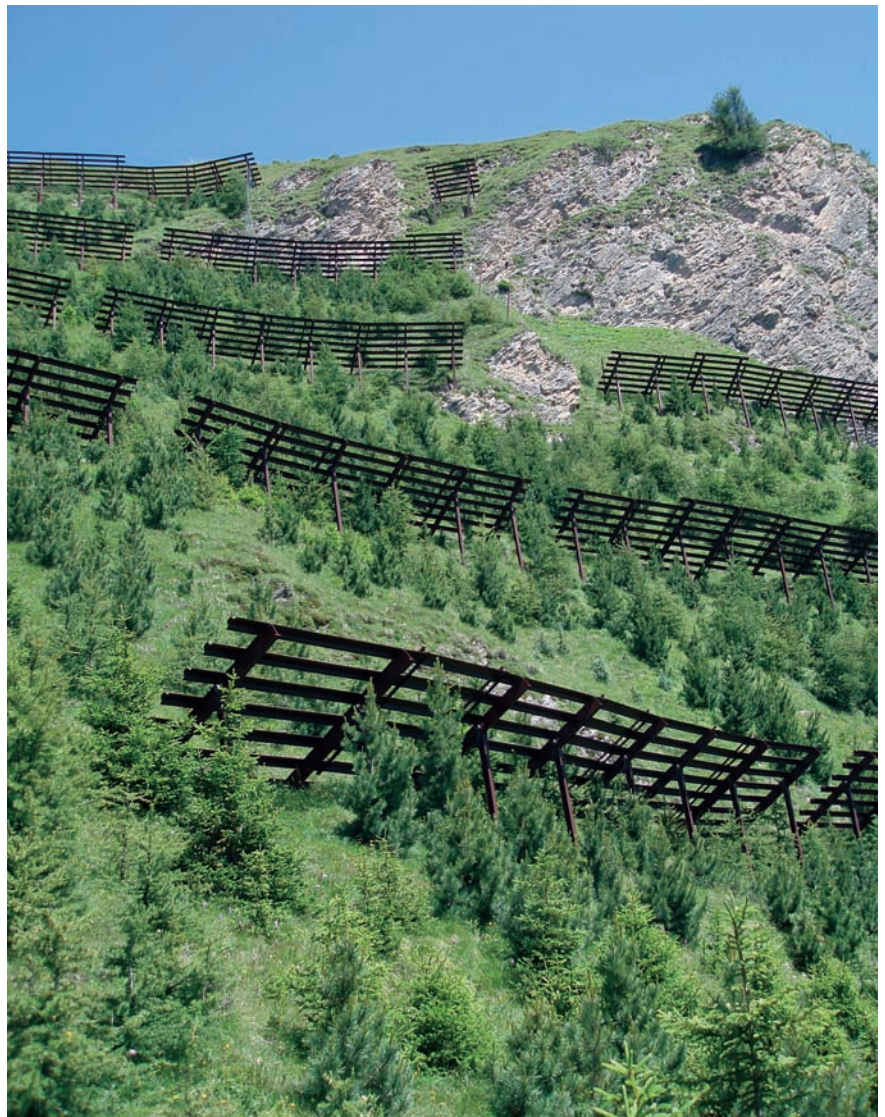
Abbildung 1: Techn. Lawinengebäuwerk mit Hochlagenaufforstung, oberhalb der Gemeinde Spiß (Tirol - Bezirk Landeck), Juli 2007
